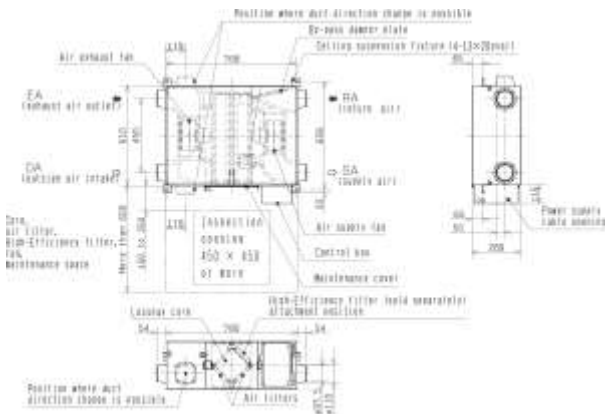
Dimensiuni LGH-15RVX-E
